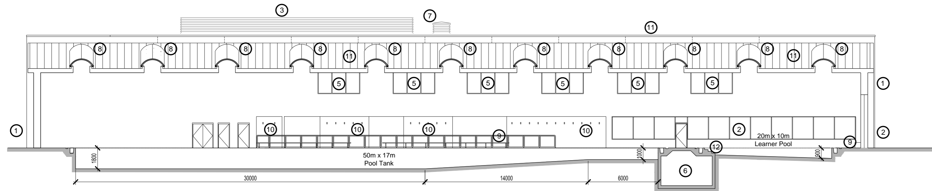
Longitudinal Section
